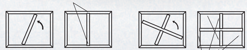
връзка кемпфер към каса mullion to frame connection
