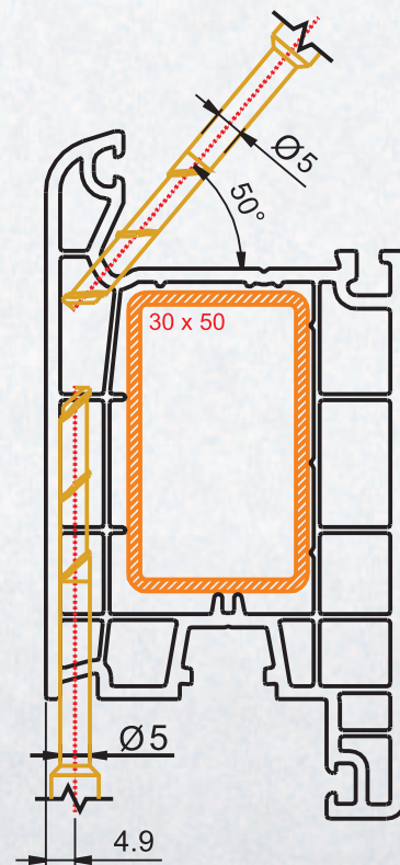
Крило врата S 538-106
