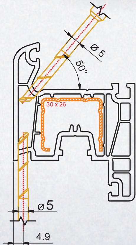
Крило прозорец S 538-103
